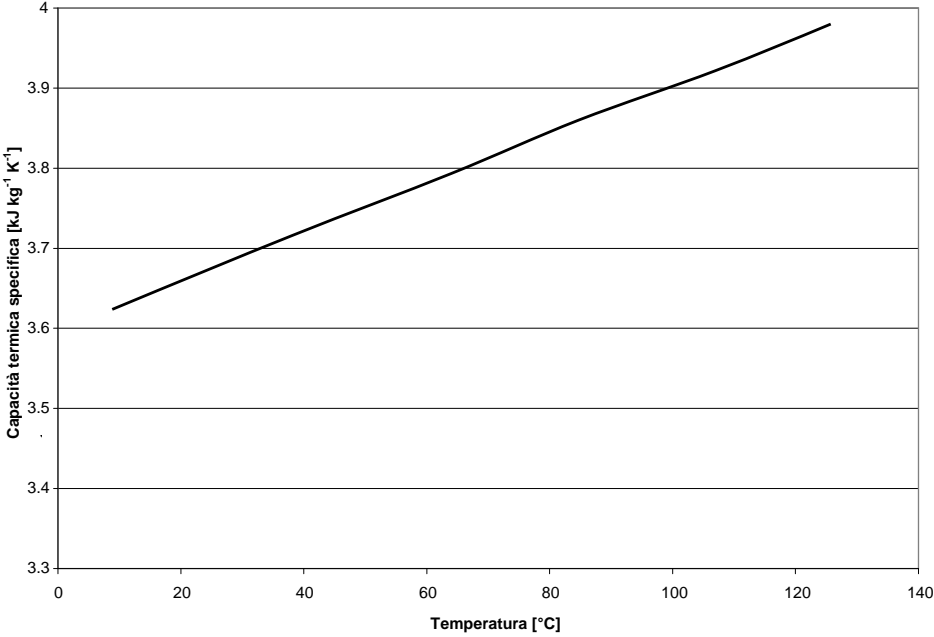
Capacità termica specifica di Fernox Solar S1
